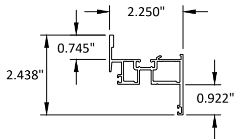
102 VENT - INSWING
