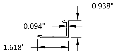
68 1" X 1 11/16" CLIP
